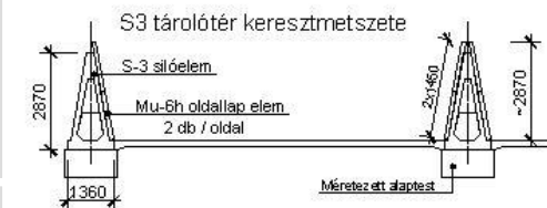
Előregyártott vasbeton silóelemekből építhető tárolótér (Keretlábak 3,00 méterenként)
