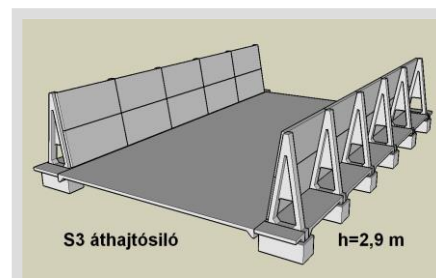
Előregyártott vasbeton silóelemekből építhető tárolótér (Keretlábak 3,00 méterenként)
