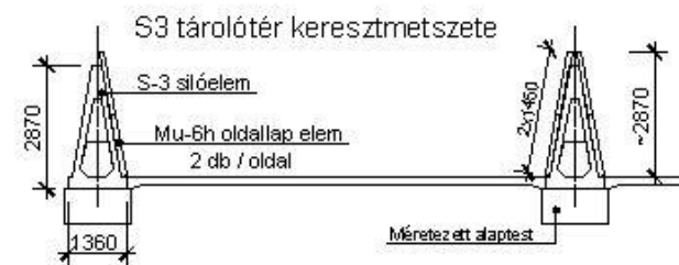
Előregyártott vasbeton silóelemekből építhető tárolótér (Keretlábak 3,00 méterenként)
