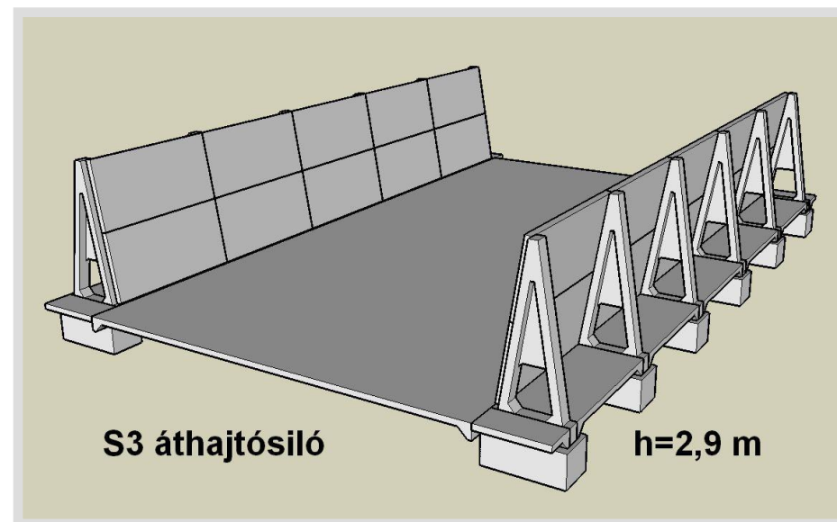
Előregyártott vasbeton silóelemekből építhető tárolótér (Keretlábak 3,00 méterenként)
