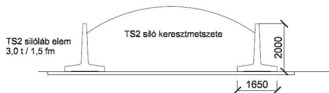
T-támfalas vasbeton silóelemekből kialakított tárolótér (Elemhossz 1,5 méter)
