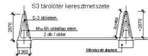
Előregyártott vasbeton silóelemekből építhető tárolótér (Keretlábak 3,00 méterenként)
